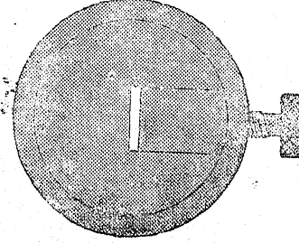
चित्र १८—शिगाफ जो रश्मि-विश्लेषक यंत्र में प्रकाश देने वाली वस्तु के सामने पड़ता है
